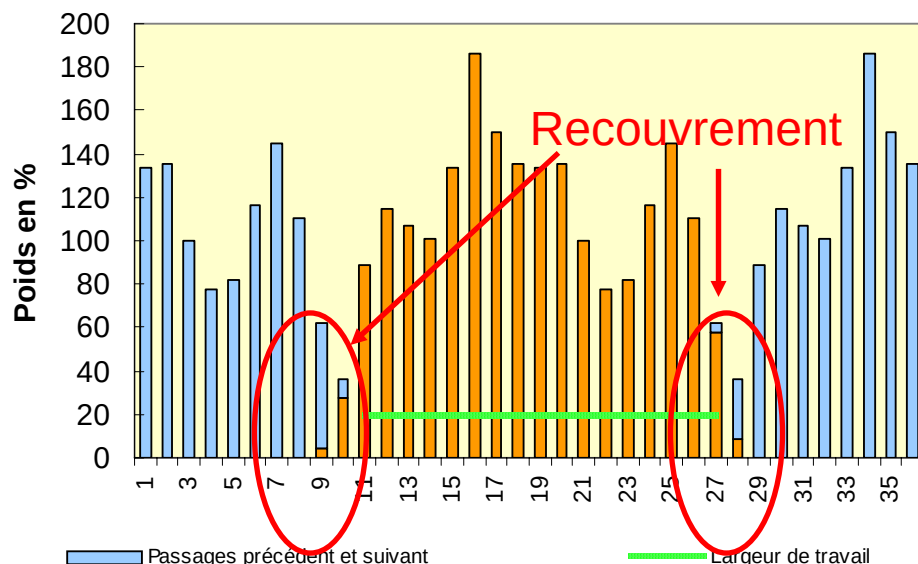
Répartition transversale : Exemple Buse à palette inversée
